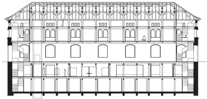
10 Der radikale Entwurf «Inversum» auf dem fünften Platz baut das Zeughaus fünfgeschossig um: Ein gespiegeltes statisches System entsteht – während die Obergeschosse an der Dachkonstruktion hängen, steht die Holzkonstruktion der Untergeschosse auf der neuen Bodenplatte. Allerdings überzeugten weder die Detailgestaltung noch der hohe Aufwand (Bild: mazzapokora, Zürich)
