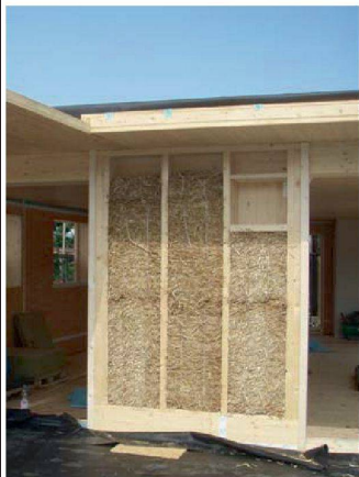
Holzbau isoliert mit Stroh
