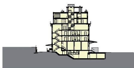
05 Schnitt A-A: Über den beiden Geschossen der Aufstockung liegt die Dachterrasse
