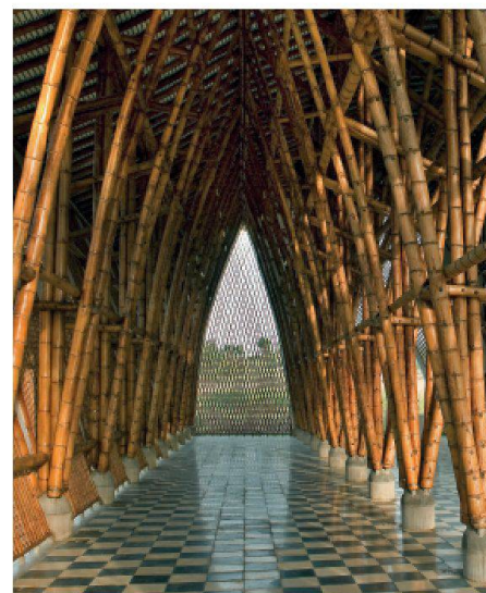
01 Die Kathedrale von Pereira, ein Temporärbau, ist gänzlich mit Guadua-Bambus ( guadua angustifolia ) konstruiert. (Foto: Deidi von Schaeuwen)
