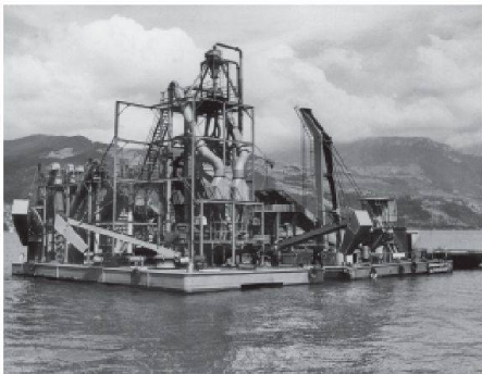
Schwimmende Tiefbaggeranlage, 1958.
