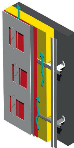
Beispielhafter Aufbau von Fassadenplatten mit lokalen, unterschiedlich geformten Öffnungen: Illustration aus dem Ventilator 4.
