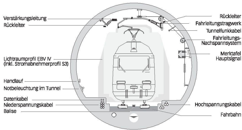
Tunnelprofil mit bahntechnischen Installationen.
