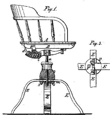
2 Patent eines Bürostuhls von Robert Fitts Jr., US Patent n. 67034, 1867 | Brevet d'une chaise de bureau de Robert Fitts Jr., US Patent n. 67034, 1867 | Brevetto di una sedia da ufficio di Robert Fitts Jr. US Patent n. 67034, 1867
