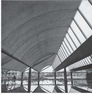
Das Sheddach des Verbands Schweizerischer Konsumvereine (VSK, heute Coop) wurde 1961 nach dem Entwurf des Ingenieurs Heinz Hossdorf erstellt. Es besteht aus Fertigteilen, die in Längsrichtung hintereinander versetzt und vorgespannt wurden. Die Konstruktion wurde damals anhand eines physischen Modells im Massstab 1:10 statisch nachgewiesen. Heute würde man dieselbe Aufgabe mit einem virtuellen Finite-Elemente-Modell (FEM) am Computer lösen.
