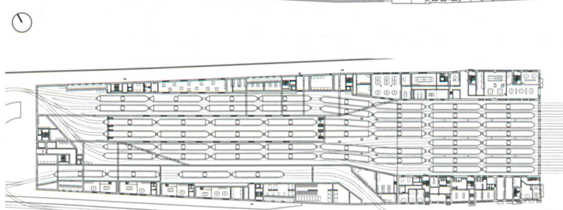
Grundriss Erdgeschoss und Regelgeschoss der Wohntürme im Mst. 1:2000.
