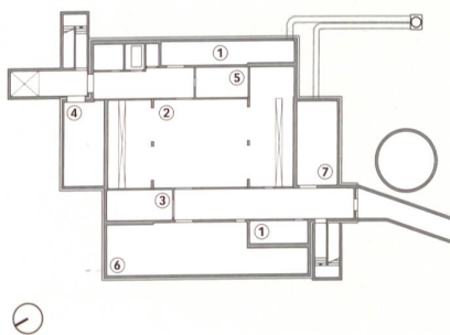
Grundriss UG.
