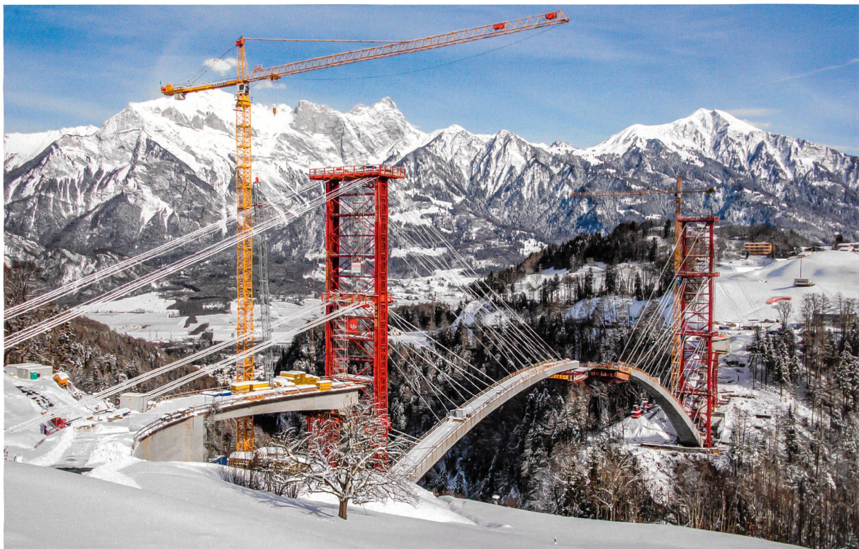
Musterbeispiel eines Freivorbauverfahrens : Bis zum Bogenschluss trug das Hilfsgerüst die auskragenden Bogenhälften.
