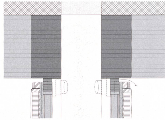
Im Detailschnitt B-B durch die Steigzone ist der Anschluss der Leichtbauwand an den Holzbalkenträger zu sehen. Kaum sichtbar ist die Luftzufuhr in den Raum über die Schattenfuge unterhalb des Holzbalkenträgers.
