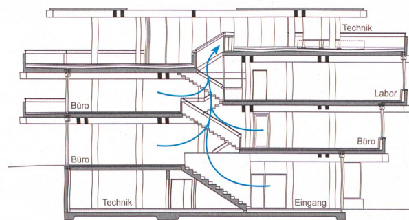
Der Schnitt A-A: Im Zentrum liegt das Atrium mit Entlüftung.
