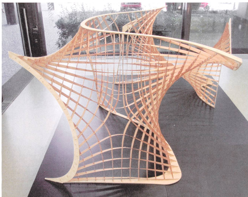
Entwurfsvorschlag für eine asymptotische Rasterschale als Pavillon (Modell): «Asymptotic Gridshell» von Denis Hitrec und Eike Schling, 2016. Die Stützstruktur wurde aus geraden Holzfurnierstreifen hergestellt. Alle Verbindungspunkte sind identisch und orthogonal.
