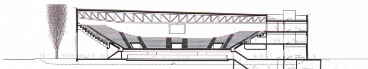
Das Siegerprojekt des Teams Frutiger in Grundriss und Schnitt, Mst. 1:1200.
