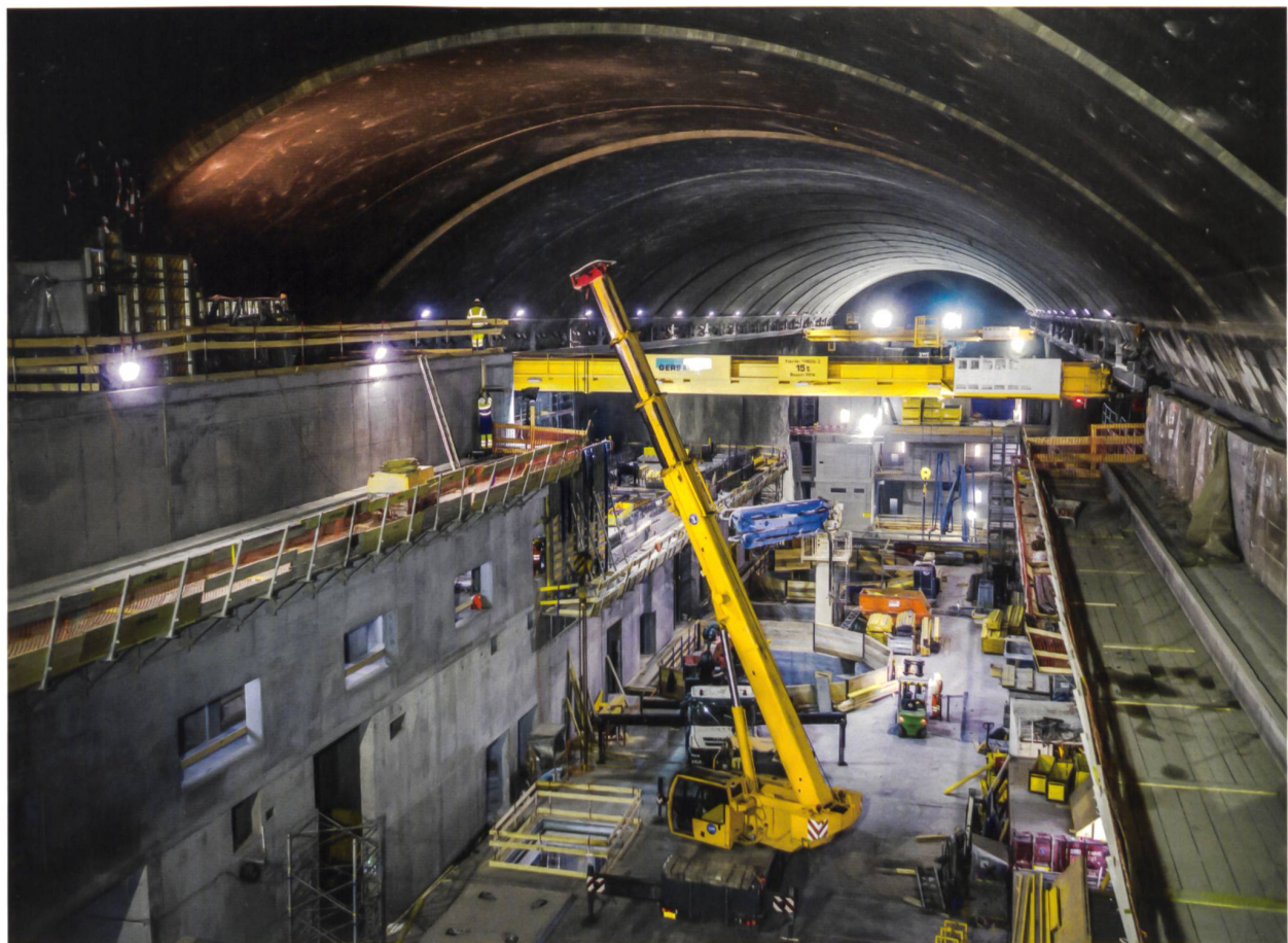
Nant de Drance: Ausbau der Maschinenkaverne. In der Bildmitte zwei der sechs Schächte für die Aufnahme der Maschinengruppen.
