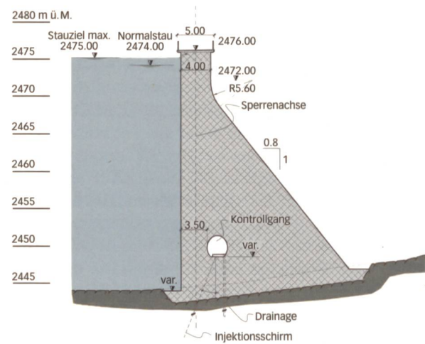
Querschnitt der Staumauer.
