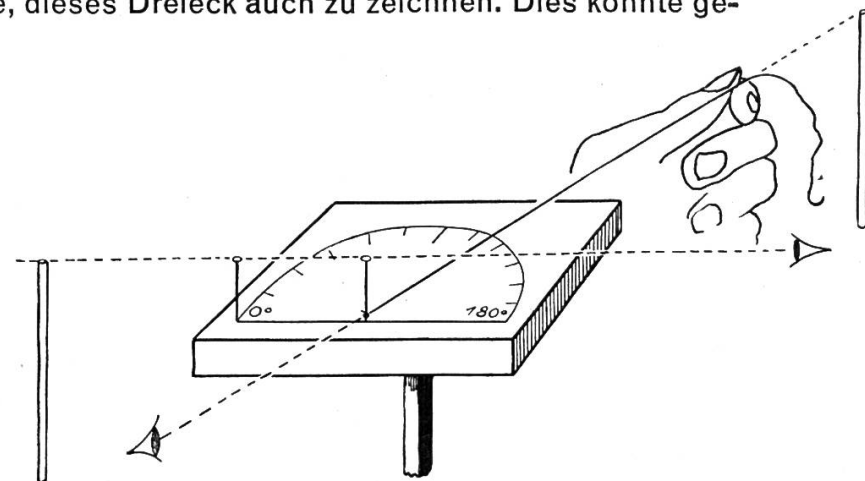
Abb. 3. Waagrechter Theodolit
