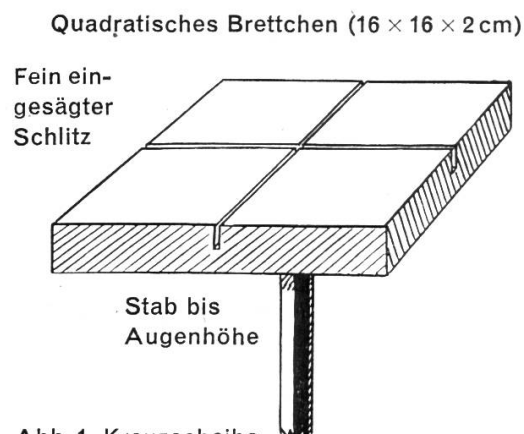
Abb. 1. Kreuzscheibe
