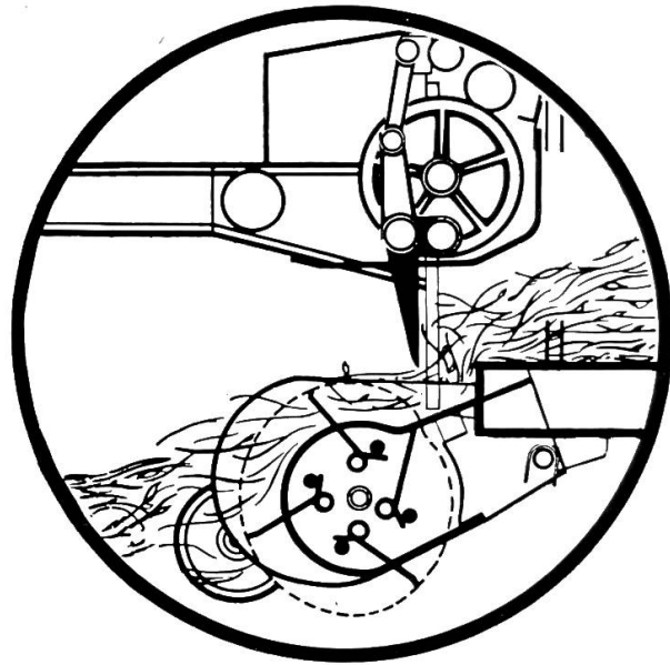
Abb. 4. Aufnahmevorrichtung eines Ladewagens: eine schnelle, rechenaubere Aufnahme von Grün- und Dörrgut jeder Art lässt sich vom Fahrzeug aus steuern
