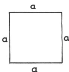
Quadrat
