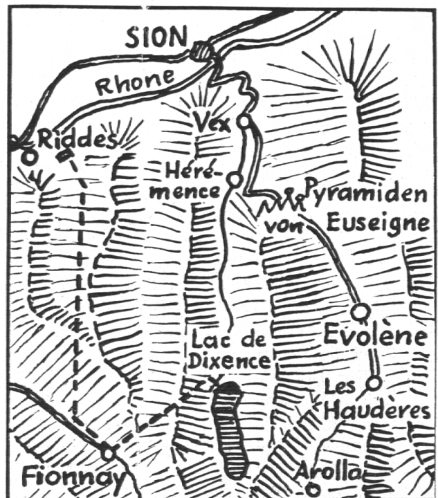
Plan der vergrößerten Kraftwerkanlage Dixence im Wallis mit künftigen Kraftwerken in Fionnay und Riddes. Der neue Staudamm wird der zweitgrößte der Welt sein (285 m hoch, 750 m lang); der Bau wird nahezu 6 Millionen m 3 Beton benötigen. Illustration zum Artikel »Die gewaltigsten Staudämme«
