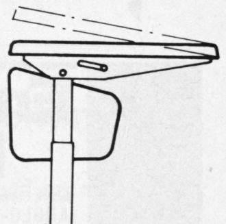
Höhenverstellung mit Klemmbolzen
