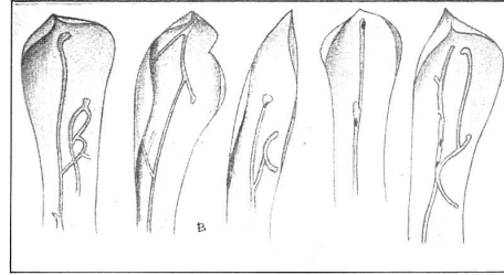
Fig. 6. Dessin de quelques galeries du type ophiomye dans les feuilles d'endive.
