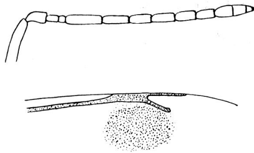
Fig. 7. — Pandelus flavipes FÖRST. ♂ : Antenne et nervulation
