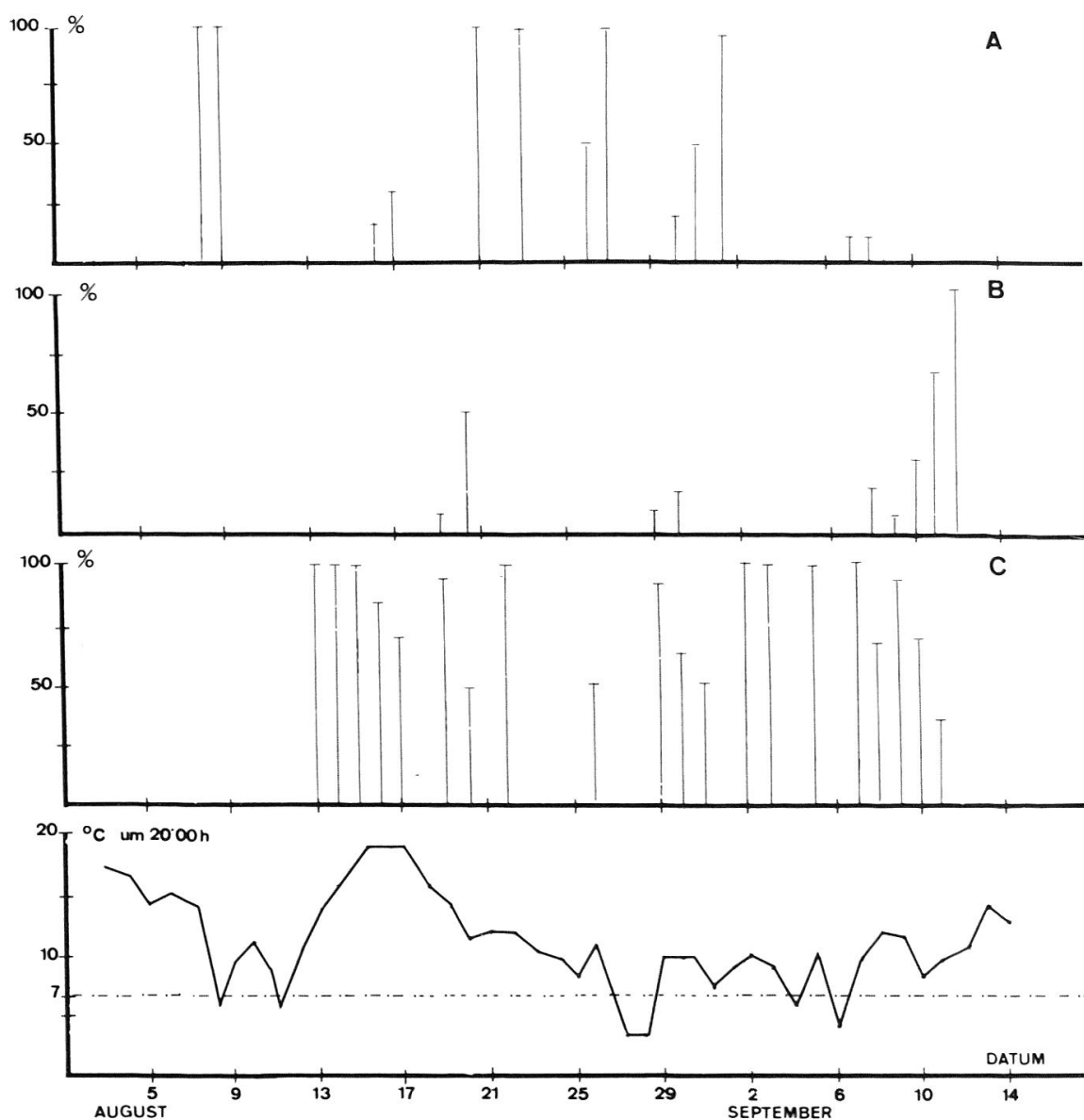
Abb. 5: Falterflug in Zuoz-Castel, 1974, nach Fangperioden getrennt (04.00-07.00 Uhr = A; 07.00-17.00 Uhr = B; 17.00-04.00 Uhr = C) (nur mit Ventilator untersucht, siehe Abb. 14).
