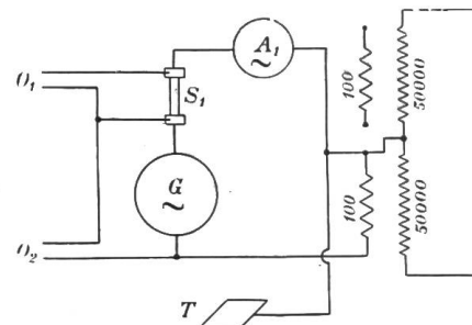
Figure 23. Schéma de la combinaison fournissant les déformations des ondes de tension et de courant de la machine révélées par les oscillogrammes A_{18} .
