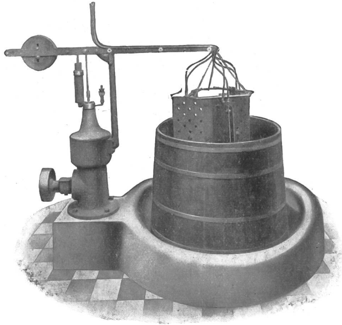
Fig. 1. Elektrischer Bremsregulator.
