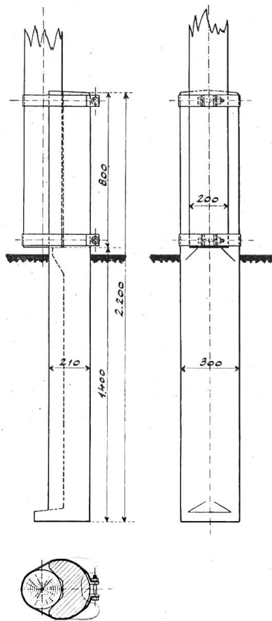
Fig. 8. Stangensockel „Universal“ Type I.
