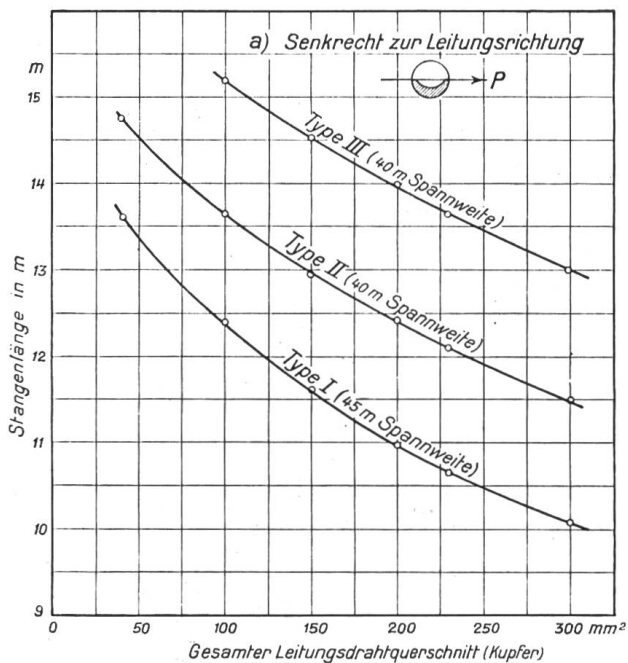
Fig. 13a. Grenzerte der Verwendbarkeit der Stangensockel „Universal“
