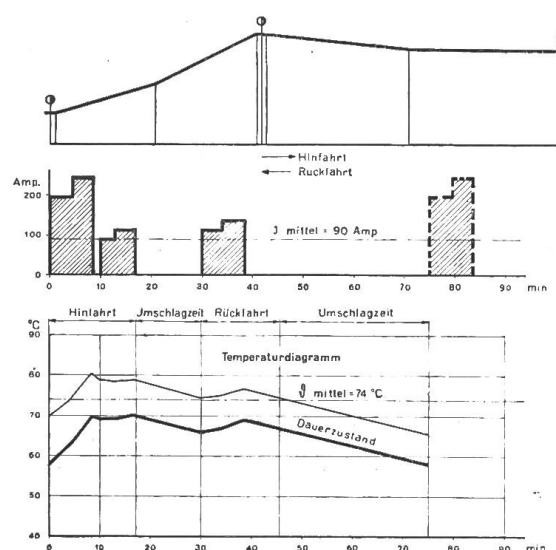
Fig. 12. Temperaturdiagramm eines Bahnmotors.
