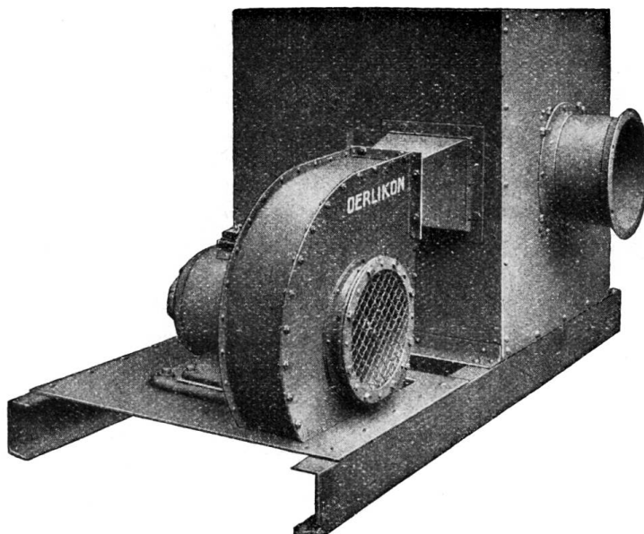
Fig. 2. Warmluftofen einer Holztrockenanlage.
