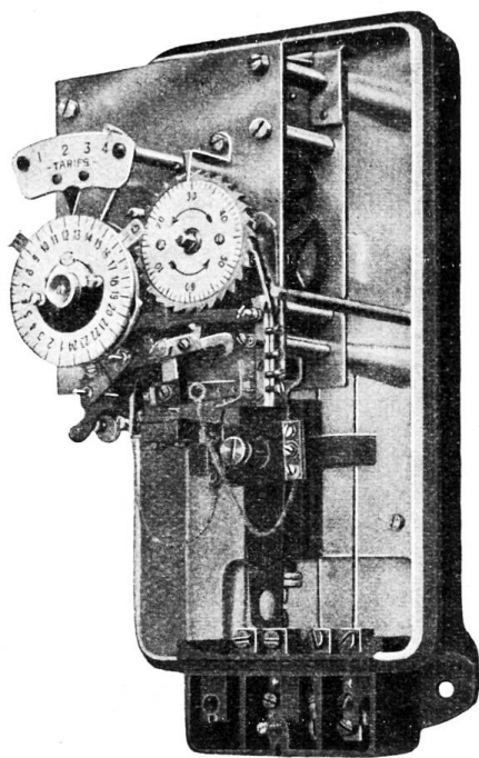
Fig. 2. Innensicht der Umschaltnur für vier Tarife.
