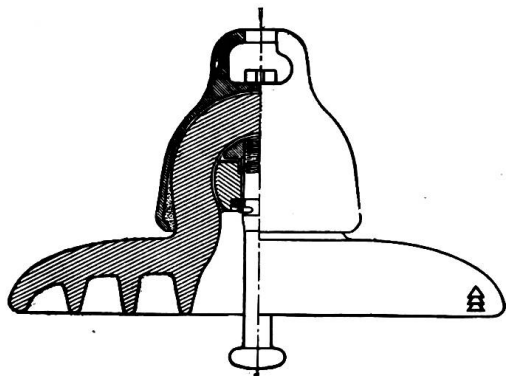
Fig. 1. Kugelpkopfisolator.
