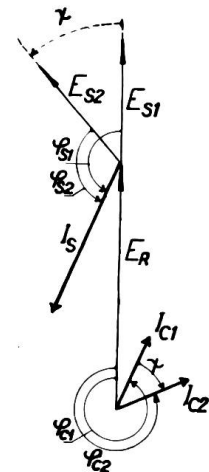
Fig. 11. Belastungsdiagramm des idealen Induktionsreglers.
