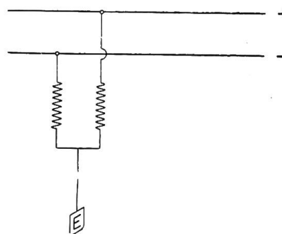
Fig. 4. Metallwiderstände zur Ableitung statischer Ladungen.
