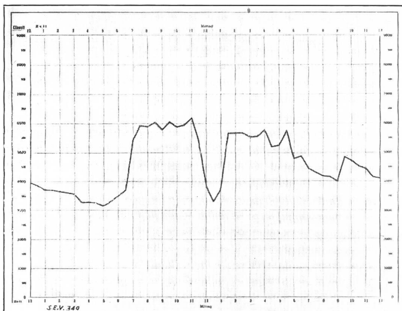
Fig. 5. Tagesbelastung des Kraftwerkes Wynau im Winter 1926.
