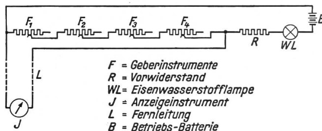
Fig. 7. Summenschialtung auf der Gleichstromseite.
