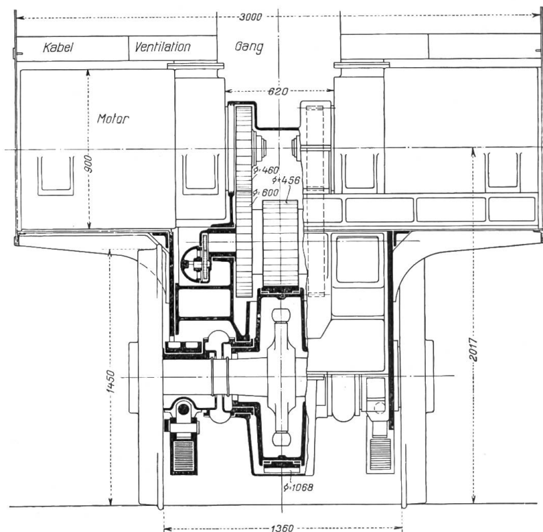
Universal-Antrieb „Winterthur“.
