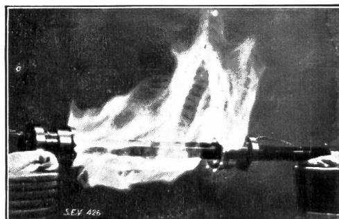
Fig. 3. „Di-EI“ Stab. Distanz = 245 mm; Ueberschlag bei 150 kV.
