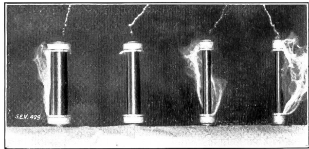
Fig. 6. Bei 120 kV (obere Grenzspannung).
