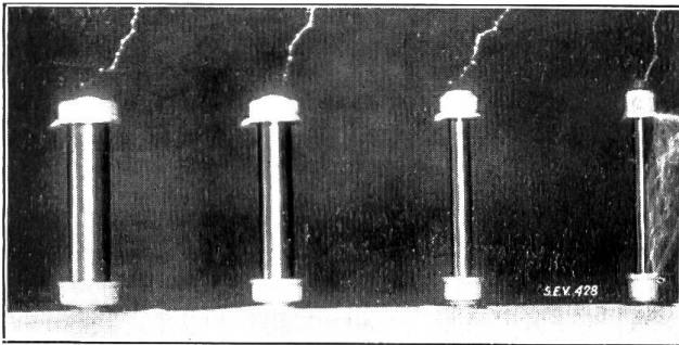
Fig. 5. Bei 117 kV (untere Grenzspannung).
