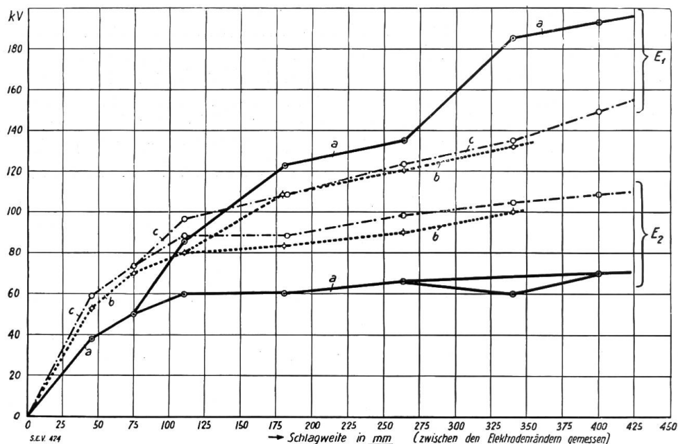
Fig. 1. Glimm- und Ueberschlagswerte an „Di-EI“ Stäben in Luft.
