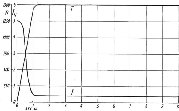
Fig. 33. Leeranlauf.
