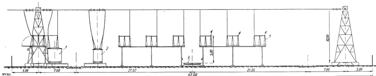
Fig. 1. Freiluft-Schaltfeld.
