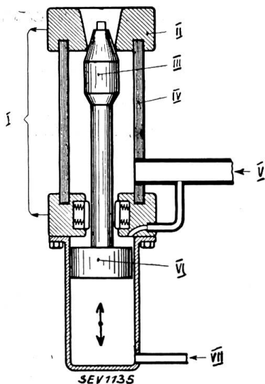
Fig. 5. Prinzipielle Skizze d. Pressluftschalters. I Elektrischer Anschluss II Fester Kontakt III Beweglicher Kontakt IV Isolationsmaterial V Pressluftzufuhr für Ausschaltstellung VI Kontaktantrieb VII Pressluftzufuhr für Einschaltstellung
