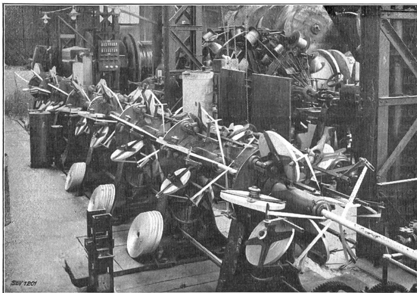
Fig. 6. Tangential-Spinner-Isoliermaschine.
