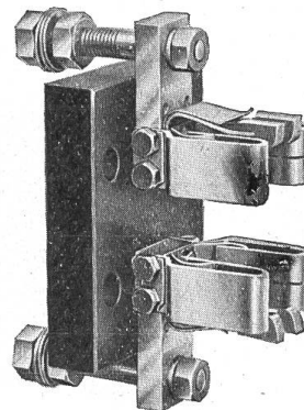
Fig. 6. Sicherungsunterteil 350 A für vorderseitigen Anschluss.
