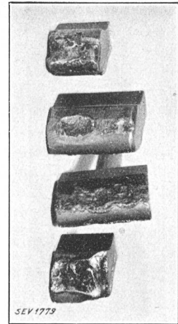
Fig. 8. Nicht kompensierte Kon- takte nach schweren Kurz- schliessungen.
