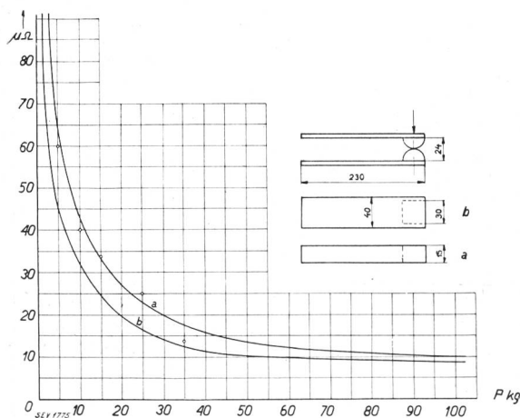
Fig. 4. Verlauf des Uebergangswiderstandes im Berührungspunkt in \mu\Omega , als Funktion des Berührungdruckes in kg bei Linearkontakten nach a und b .
