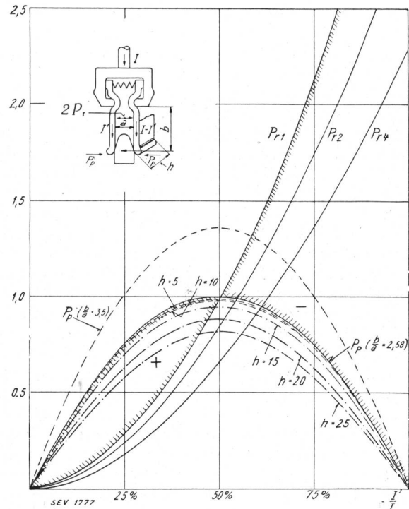
Fig. 6. Anziehungskräfte P_p und Repulsionskräfte P_r in 100% in Funktion der Stromunsymmetrie \frac{I'}{I} .
