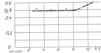
Fig. 17. tg δ-Charakteristik der ganzen Wicklung eines Generators von 16 800 kW, 10 500 V, ausgerüstet mit Asphaltmikanit-isolierung.
