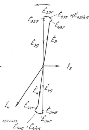
Fig. 7. Vollständiges Vektordiagramm der läufererregten kommutierten Maschine.
