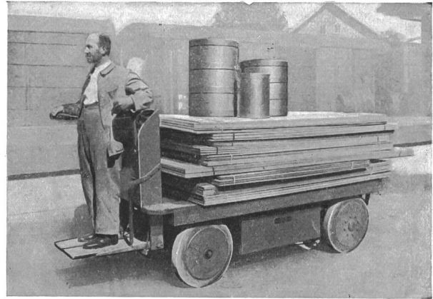
Fig. 17. Elektrokarren. Nutzlast 2000 kg.
