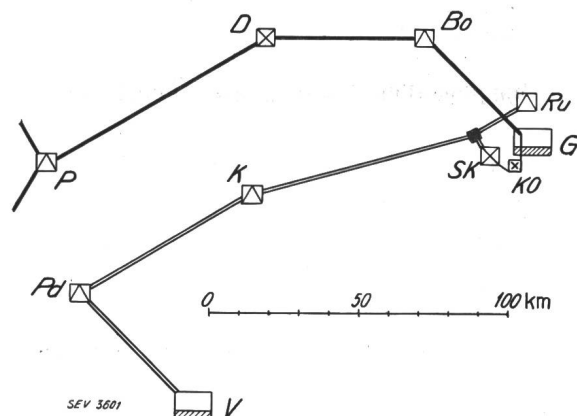
Fig. 5. Lageplan der im Jahre 1933 beobachteten Netze. System A der Fig. 6 (80 kV). System B (132 kV).
