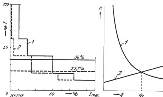
Fig. 1. Jahresbelastungsdiagramm einer Anlage mit 3160 «Benutzungsstunden» bei 1990 «Verluststunden» ( f_v = 22,7 Prozent). 1 Belastungsdiagramm. 2 Verlustdiagramm (Maßstab 100 mal kleiner).
