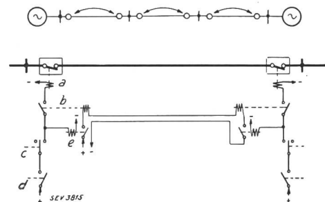
Fig. 3. Streckenschutz für zweiseitig gespeiste Leitungen. a Auslöser. b Vergleichsfreigaberrelais. c Richtungsrelais. d Anregereleais. e Steuerfreigaberrelais.
